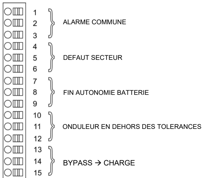
Illustration 11 – Bornes de la carte relais
