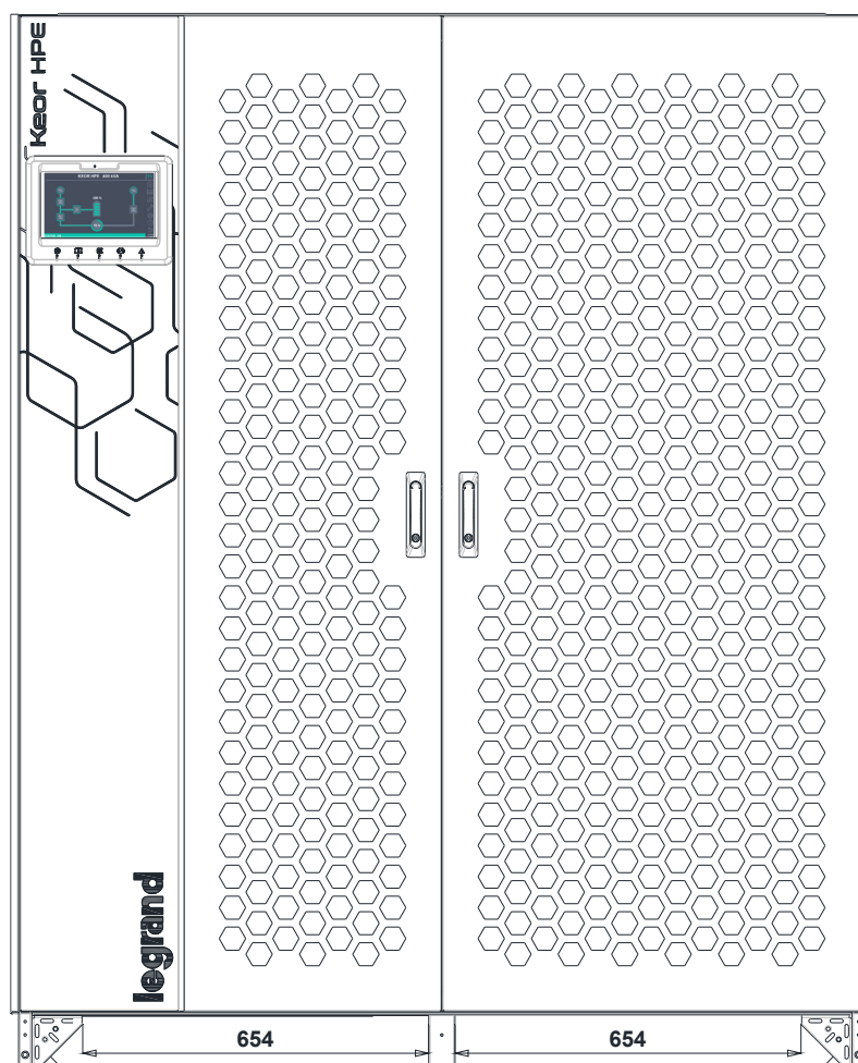
Figura 2A – Movimentazione UPS KEOR HPE 600 kVA
