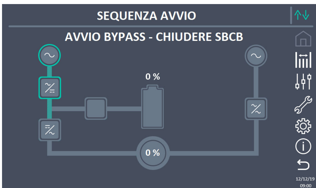
Figura 15 – Avvio bypass
