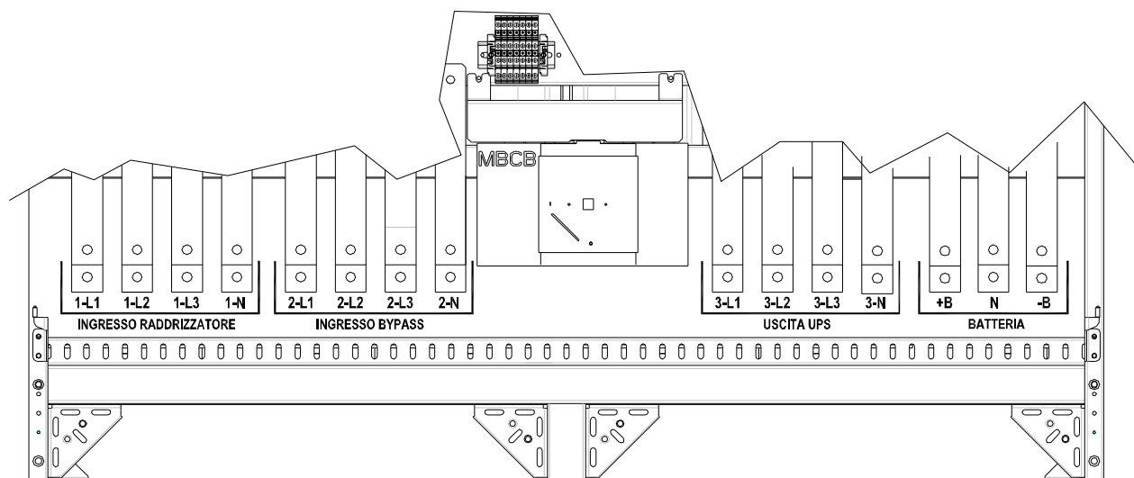
Figura 8A – Morsettiera KEOR HPE 400-500 kVA
