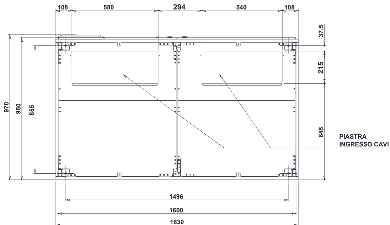
Figura 3A – Pianta di base KEOR HPE 600kVA
