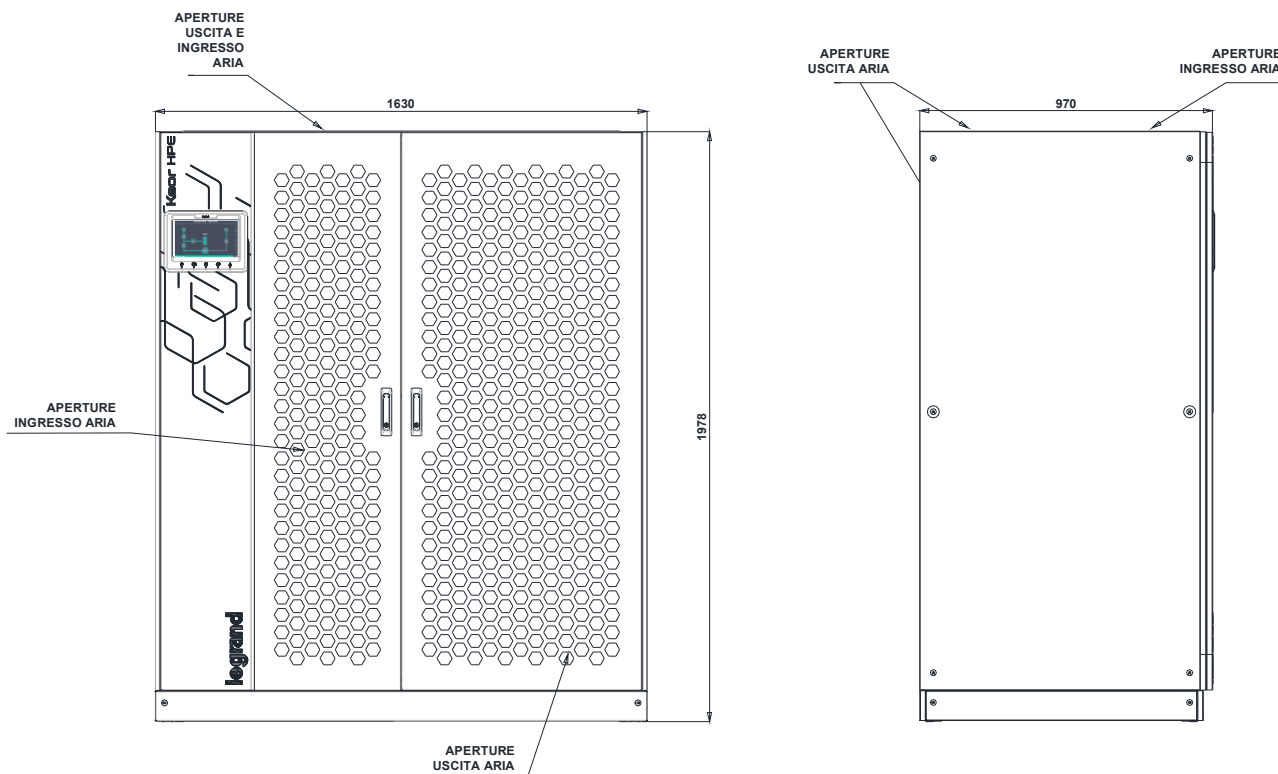
Figura 4A – Dimensioni di ingombro KEOR HPE 600kVA
