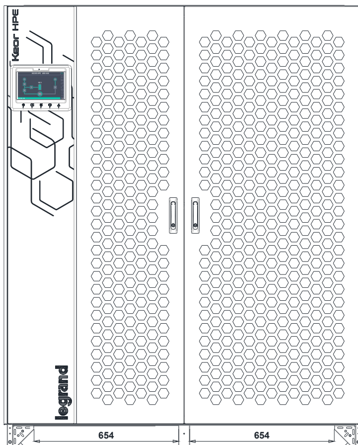
Illustration 2A – Manutention de l'ASI KEOR HPE 600 kVA
