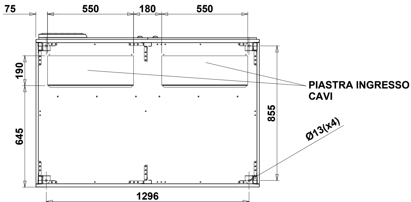
Figura 3 – Pianta di base KEOR HPE 400-500kVA
