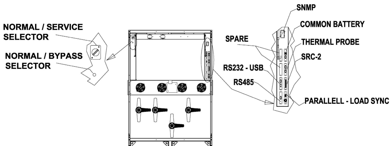
Figura 10 – Posizione schede di interfaccia KEOR HPE 400-500kVA
