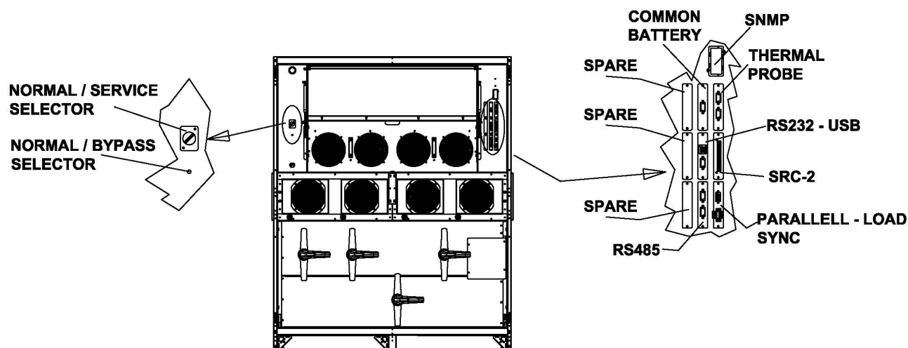
Illustration 10A – Position des interfaces de série du KEORHPE 600 kVA
