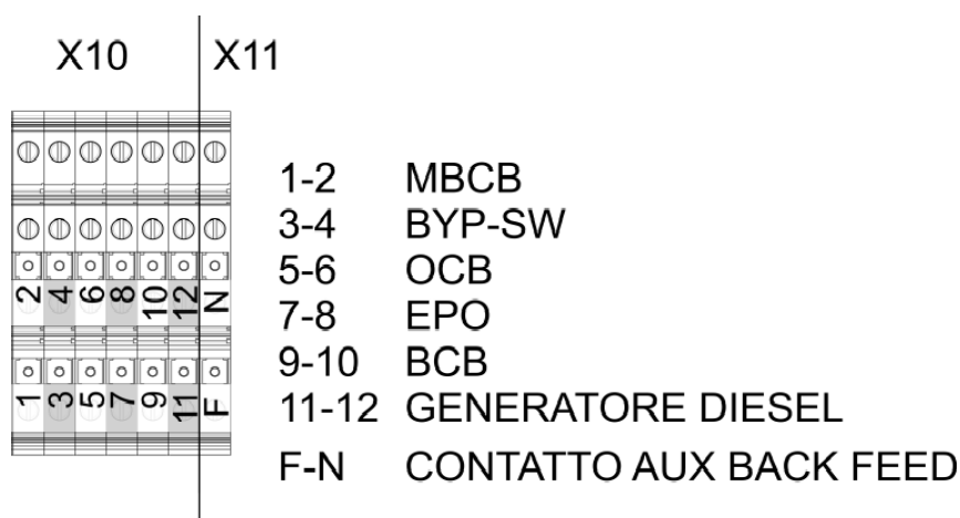
Illustration 9 – Bornes auxiliaires du KEOR HPE 400-500 kVA
