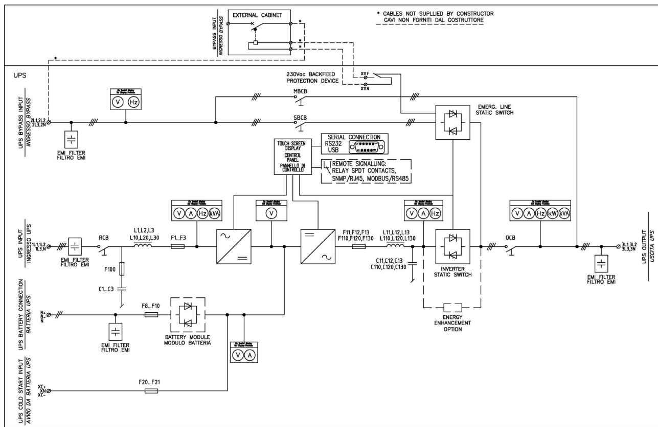
Figura 8 – Schema unifilare KEOR HPE 400-500-600 kVA con collegamento al dispositivo esterno
