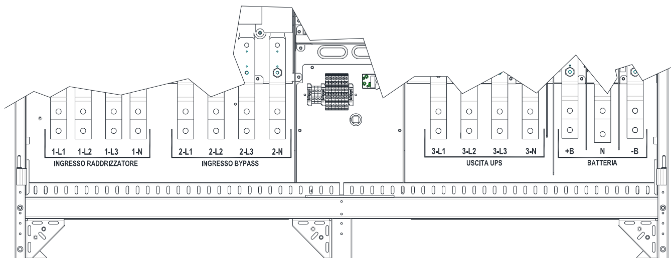
Figura 8B – Morsettiera KEOR HPE 600 kVA
