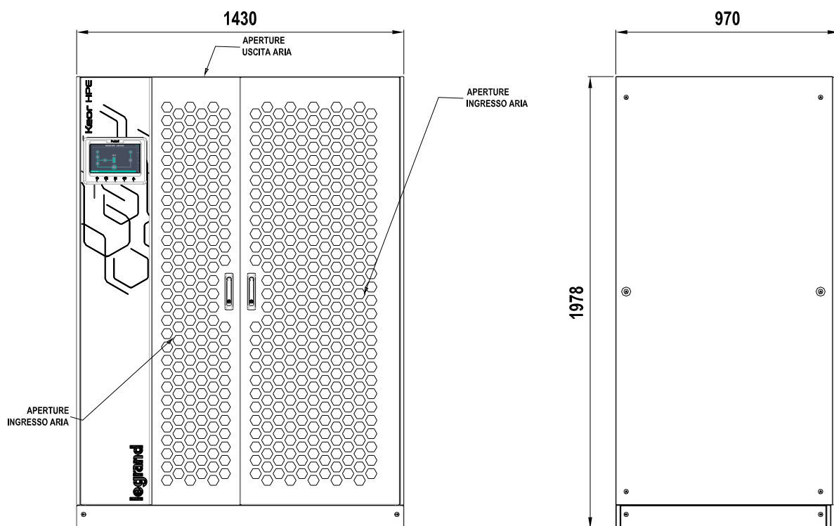
Figura 4 – Dimensioni di ingombro KEOR HPE 400-500kVA
