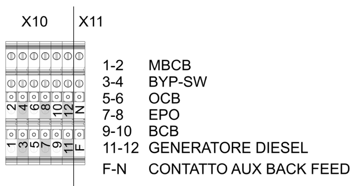
Figura 9 – Morsetti ausiliari KEOR HPE 400-500 kVA
