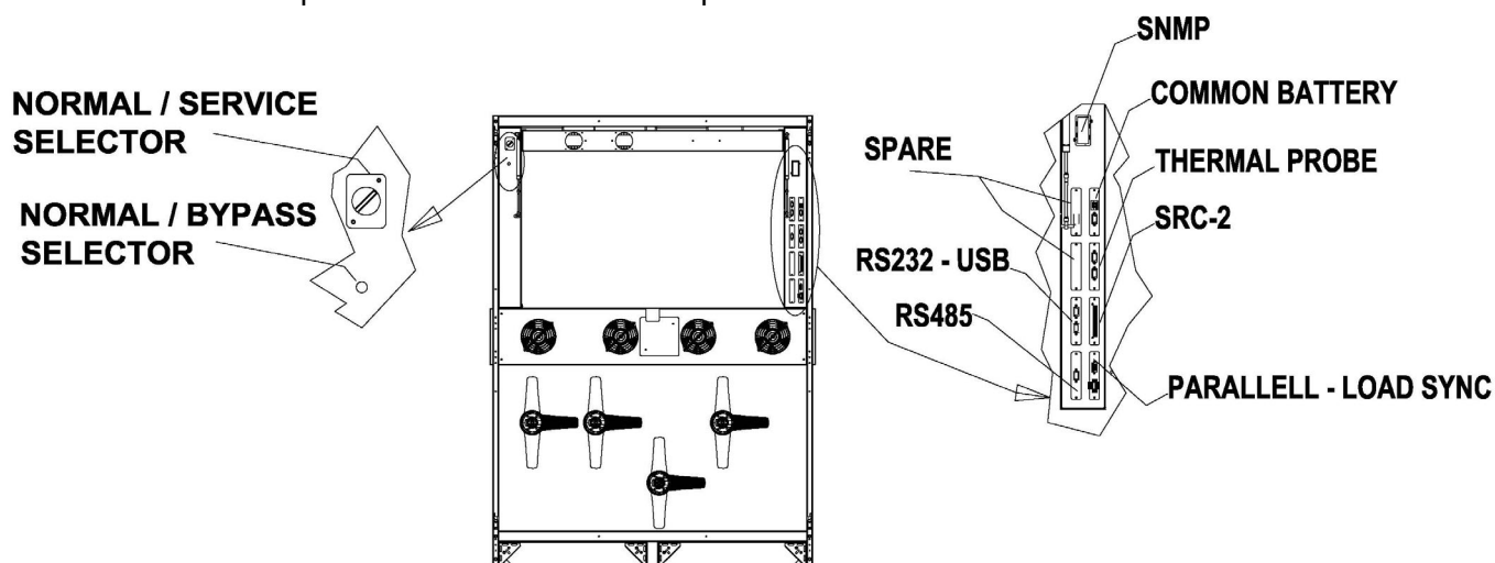
Illustration 10 – Position des interfaces de série du KEORHPE 400-500 kVA
