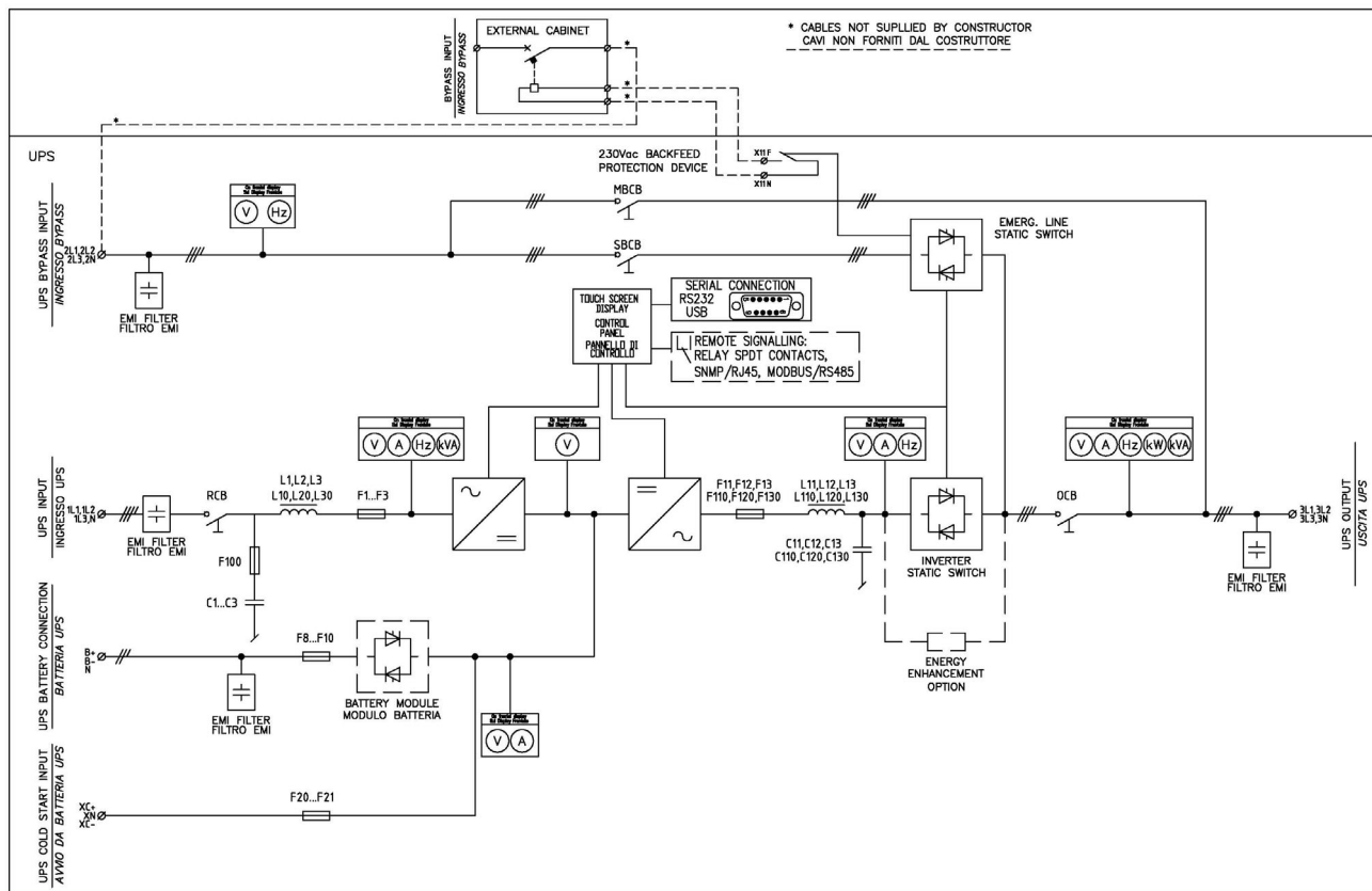
Illustration 8 – Diagramme à une ligne KEOR HPE 400-500-600 kVA avec connexion à un périphérique externe
