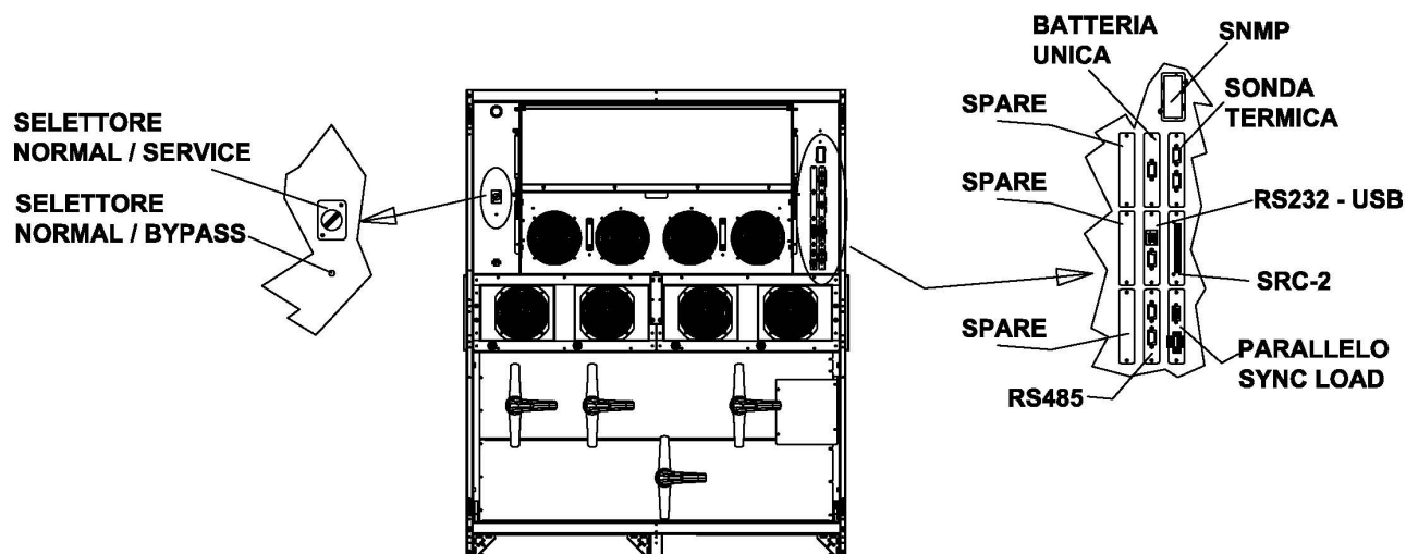
Figura 10A – Posizione schede di interfaccia KEOR HPE 600kVA
