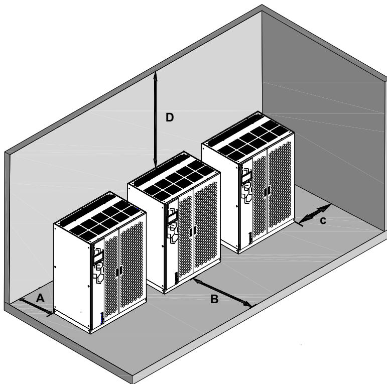
Illustration 5 – Dégagement minimum
