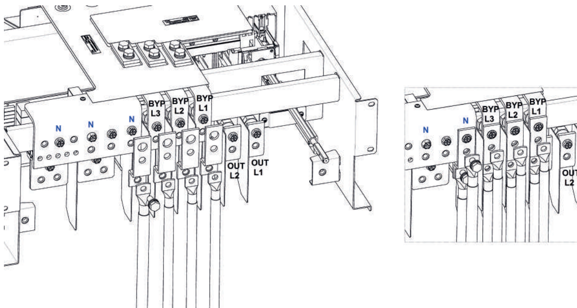
KEOR MOD 125 - installazione cavi di bypass con accessori per cavo doppio e linea di ingresso separata dalla linea di bypass
