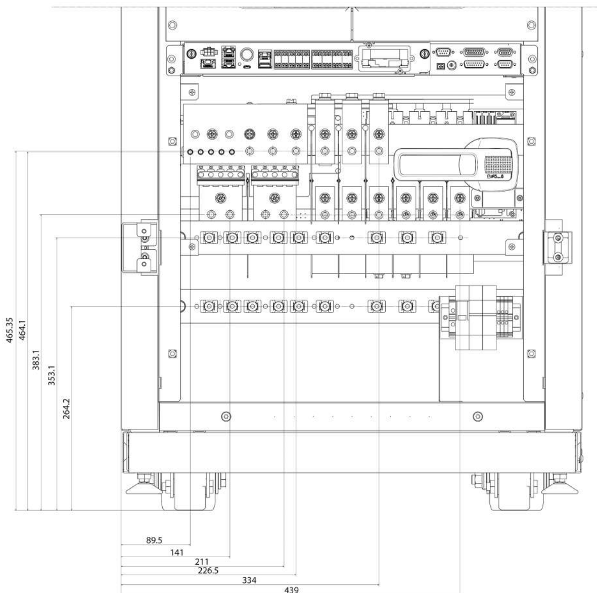
KEOR MOD 125 – vista delle due barre metalliche per ancoraggio cavi
