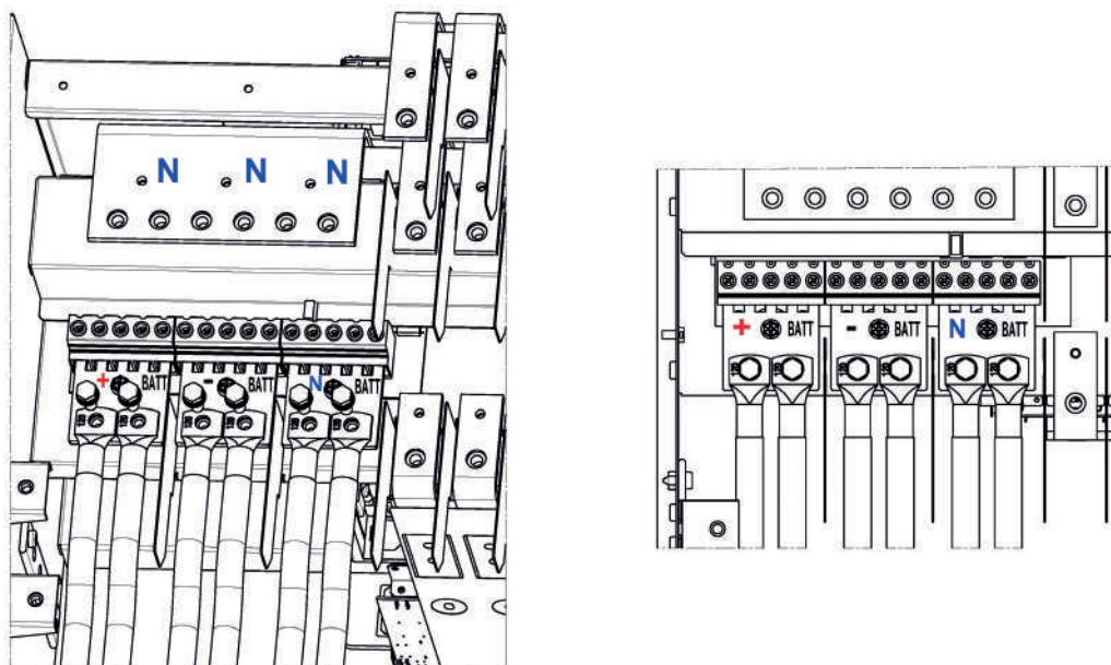
KEOR MOD 250 – installazione dei cavi di batteria con stringhe di batterie in comune (cavo doppio)
