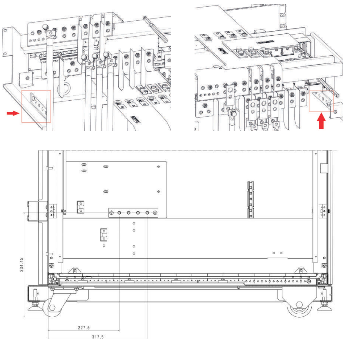
KEOR MOD 125 – barre di messa a terra
