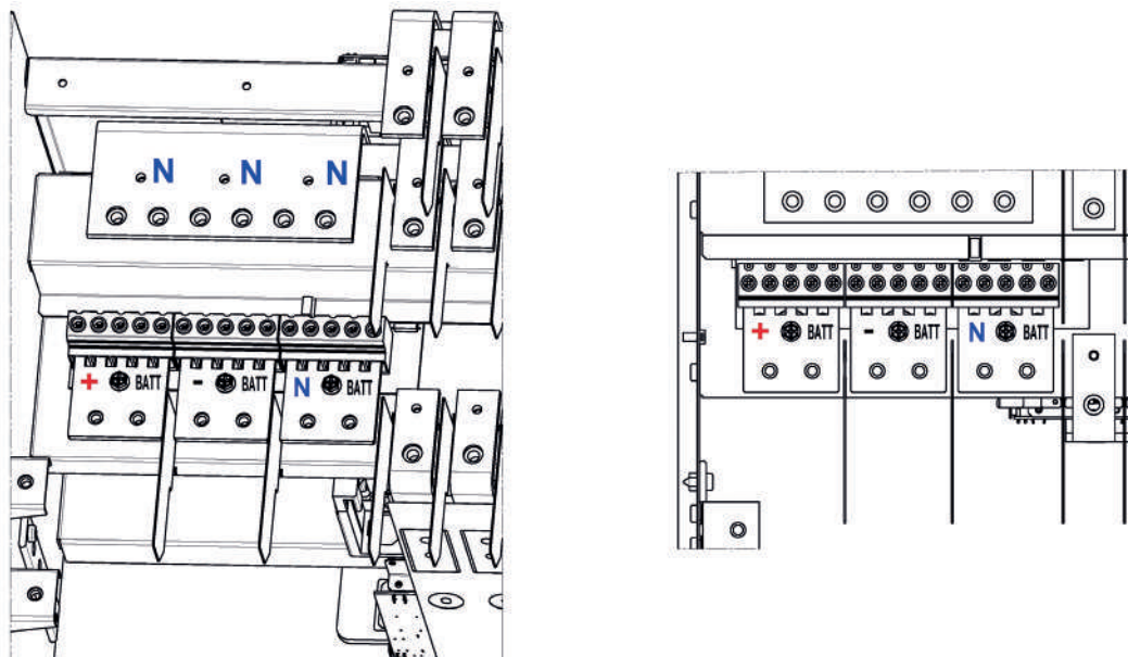
KEOR MOD 250 – morsetti di batteria
