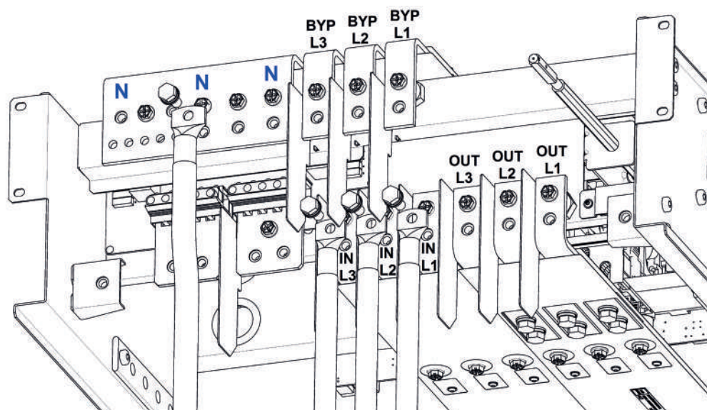
KEOR MOD 125 – installazione cavi di ingresso con linea di ingresso separata dalla linea di bypass
