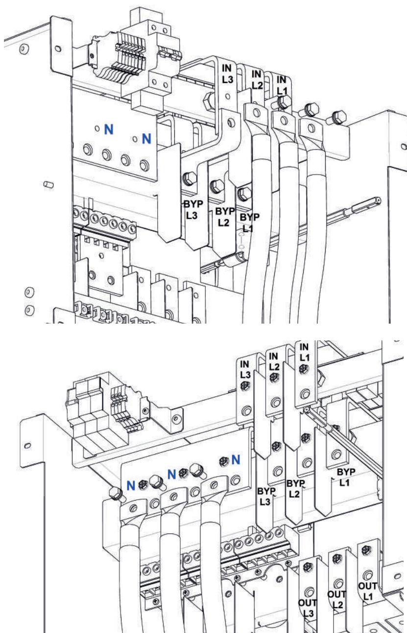
KEOR MOD 250 - installazione cavi di ingresso con linea di ingresso in comune con linea di bypass
