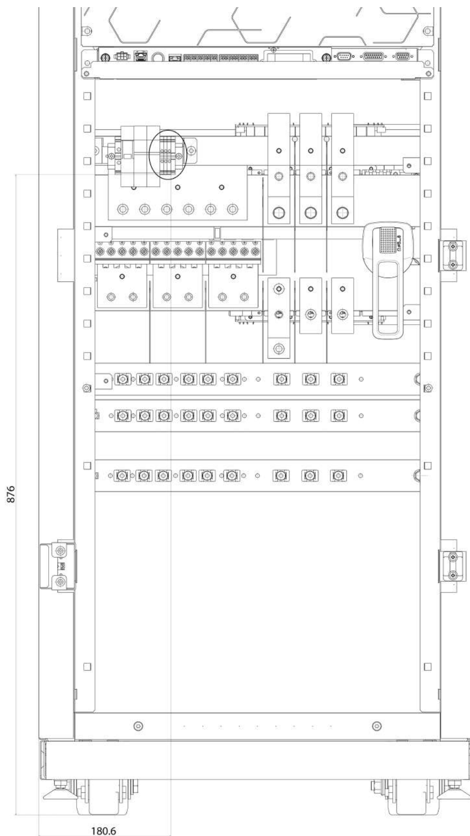
KEOR MOD 250 – vista delle tre barre metalliche per ancoraggio cavi
