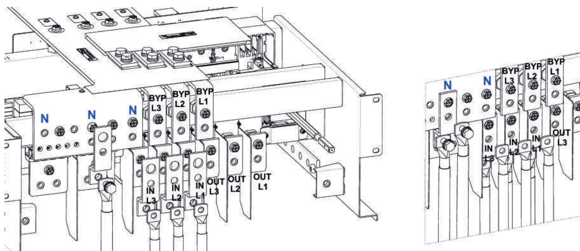
KEOR MOD 125 - installazione cavi di ingresso con accessori per cavo doppio e linea di ingresso separata dalla linea di bypass
