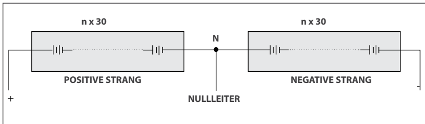
Zwei in Reihe geschaltete Batteriestränge mit Mittelabgriff – Nullleiterpotenzial –
