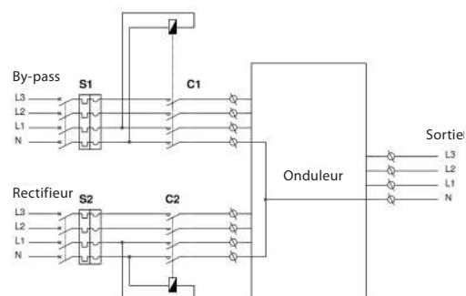
Entrée Double Systèmes TT/TNS
