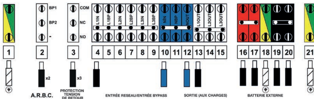
Trimod MCS 30 avec ligne d'entrée bypass commune
