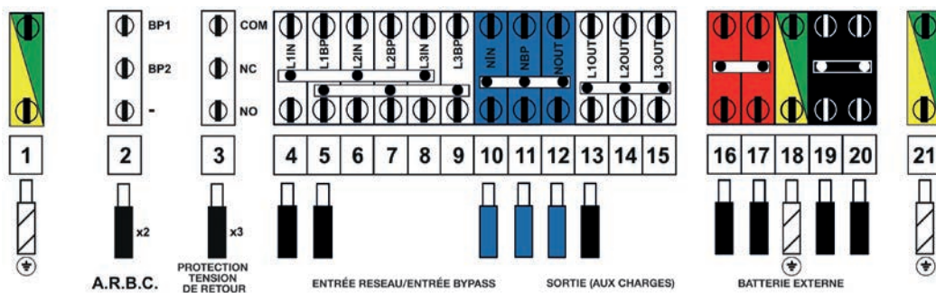
Trimod MCS 30 avec ligne d'entrée bypass séparée
