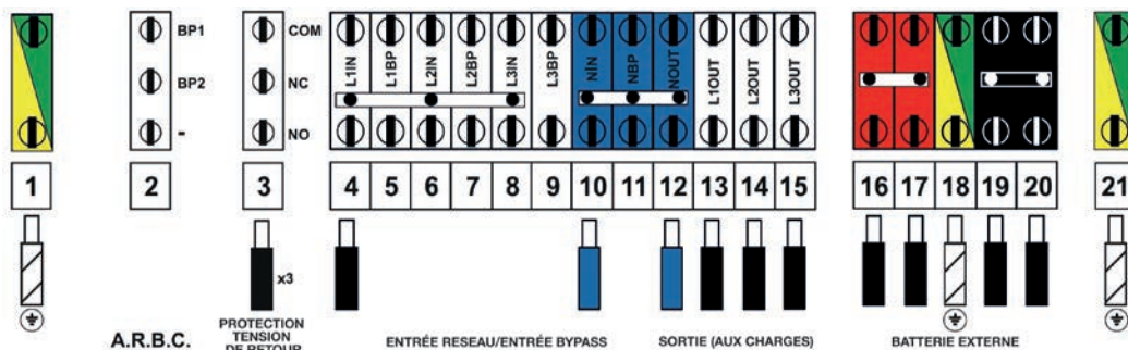
Trimod MCS 30 (avec ligne d'entrée bypass désactivée)
