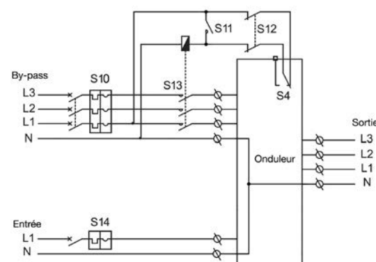
Configuration Monophasé/Triphasé
