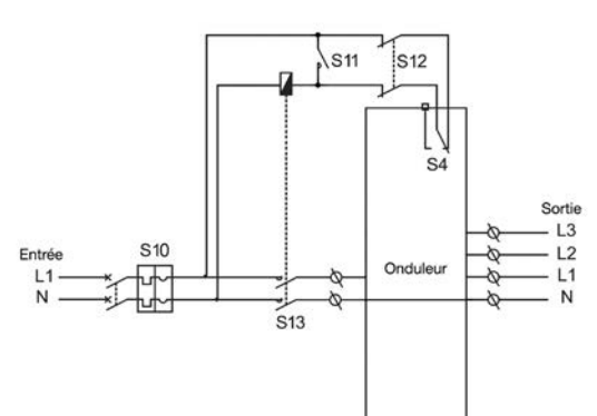
Configuration Monophasé/Triphasé
