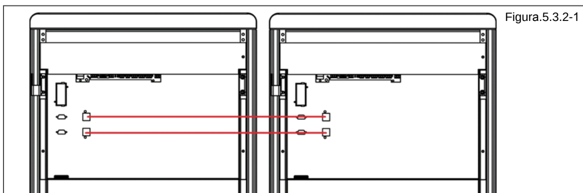
CONEXIÓN CANBUS DE DOS SAI EN PARALELO
