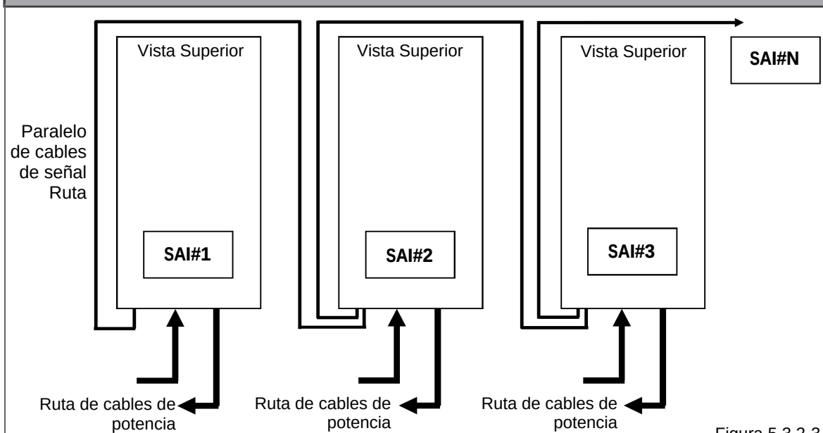
CONEXIÓN CANBUS DE TRES O MÁS SAI EN PARALELO
