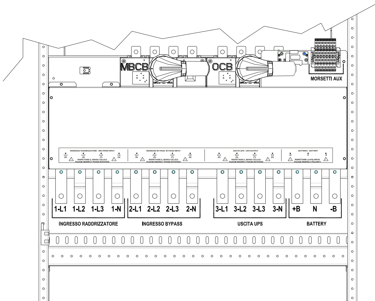
Figura 6A – Morsettiera KEOR HPE 300 kVA
