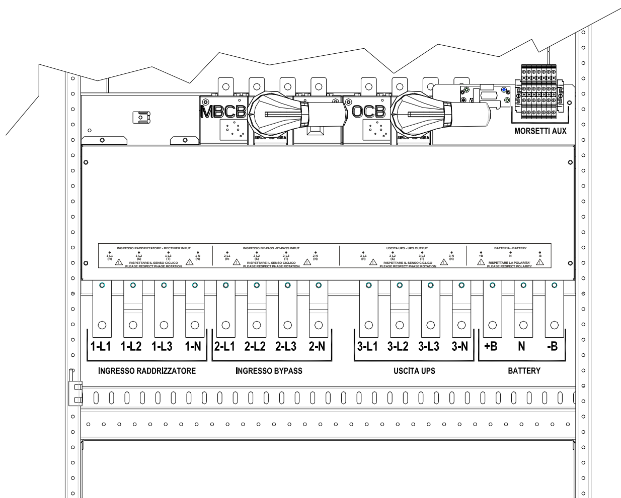
Figura 6 – Morsettiera KEOR HPE 200-250 kVA
