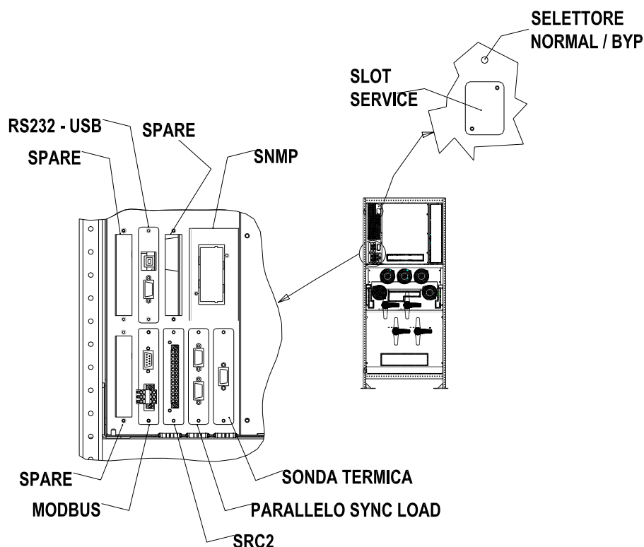
Figura 8 – Posizione schede di interfaccia KEOR HPE 200-250-300kVA
