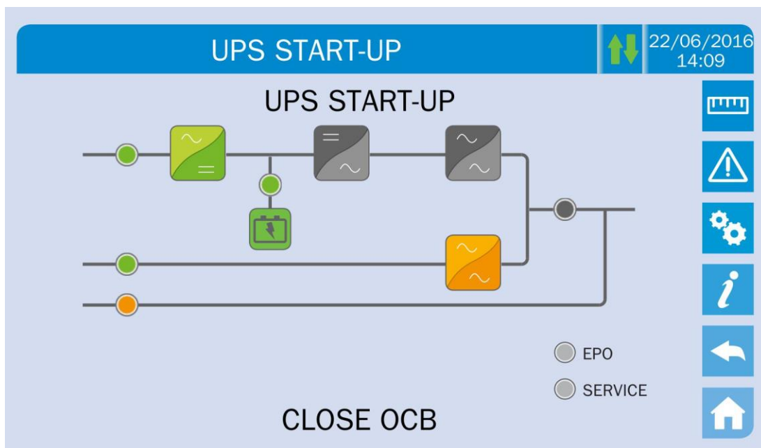
Illustration 20 – Fermeture de l'interrupteur de sortie de l'onduleur
