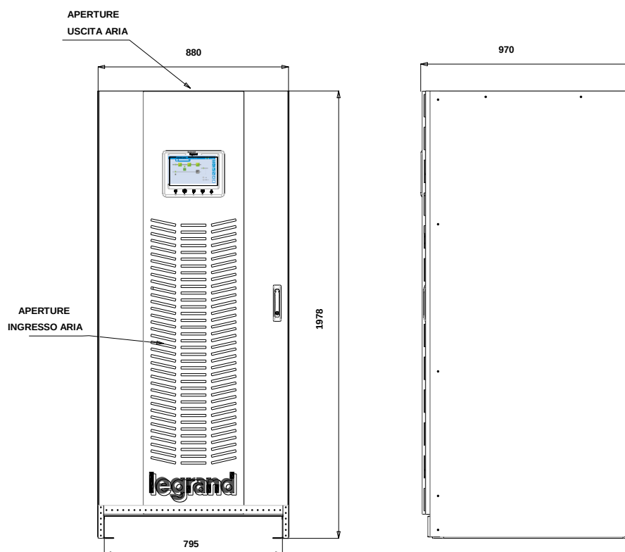
Figura 4 – Dimensioni di ingombro
