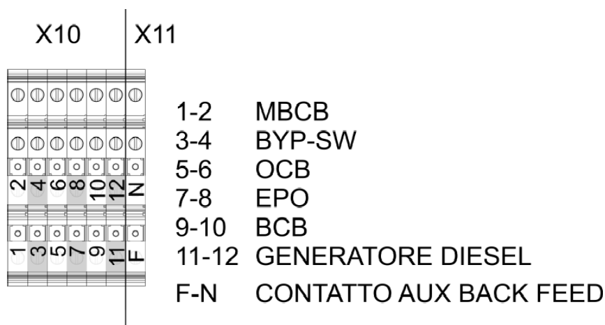
Illustration 7 – Bornes auxiliaires du KEOR HPE 200-250-300 kVA
