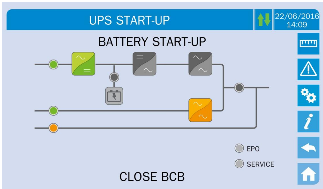
Illustration 19 – Connexion de la batterie
