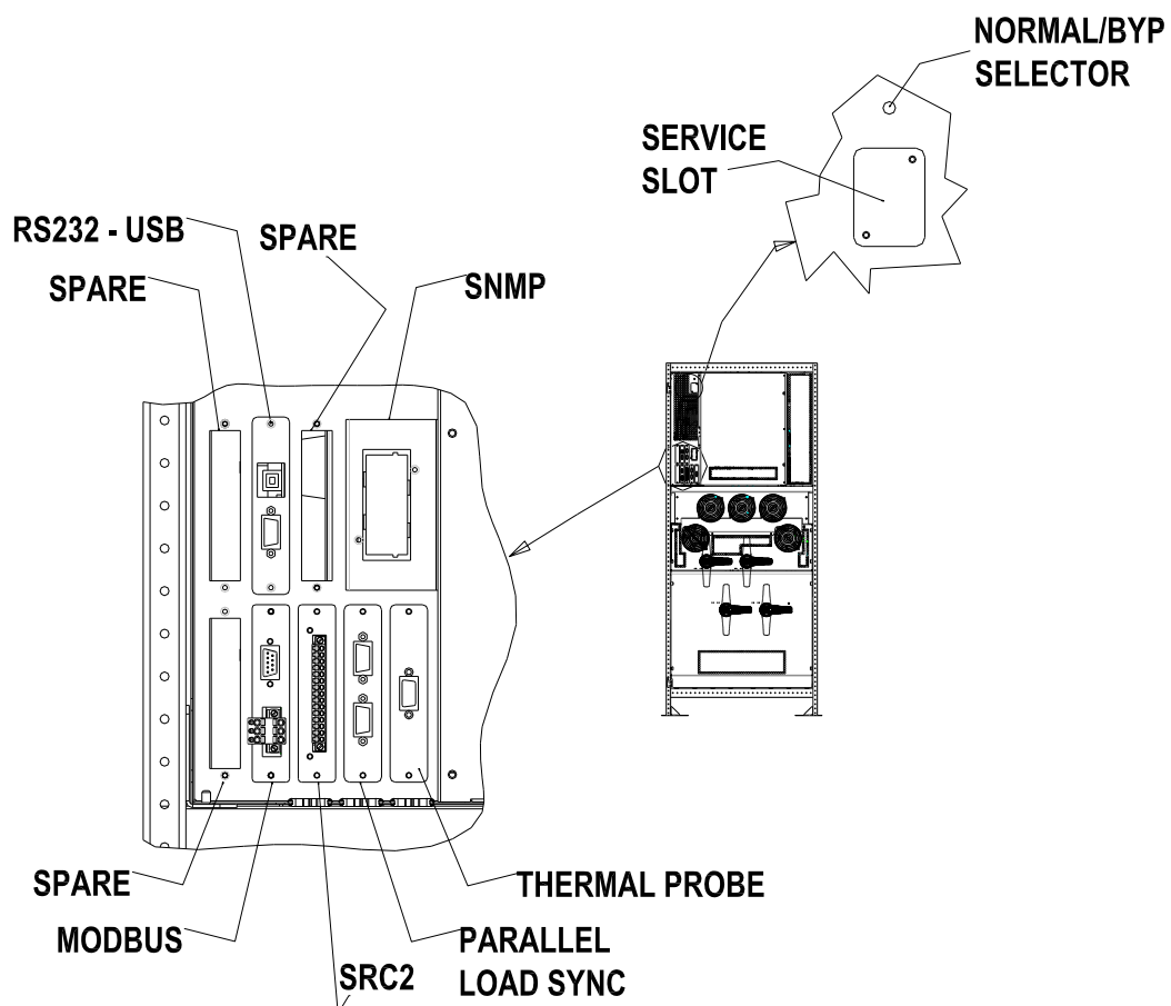
Illustration 8 – Position des interfaces de série du KEORHPE 200-250-300 kVA
