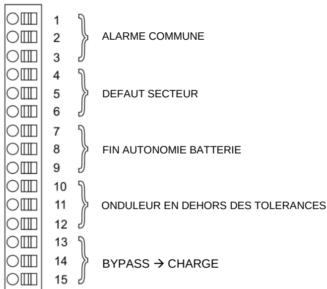
Illustration 9 – Bornes de la carte relais
