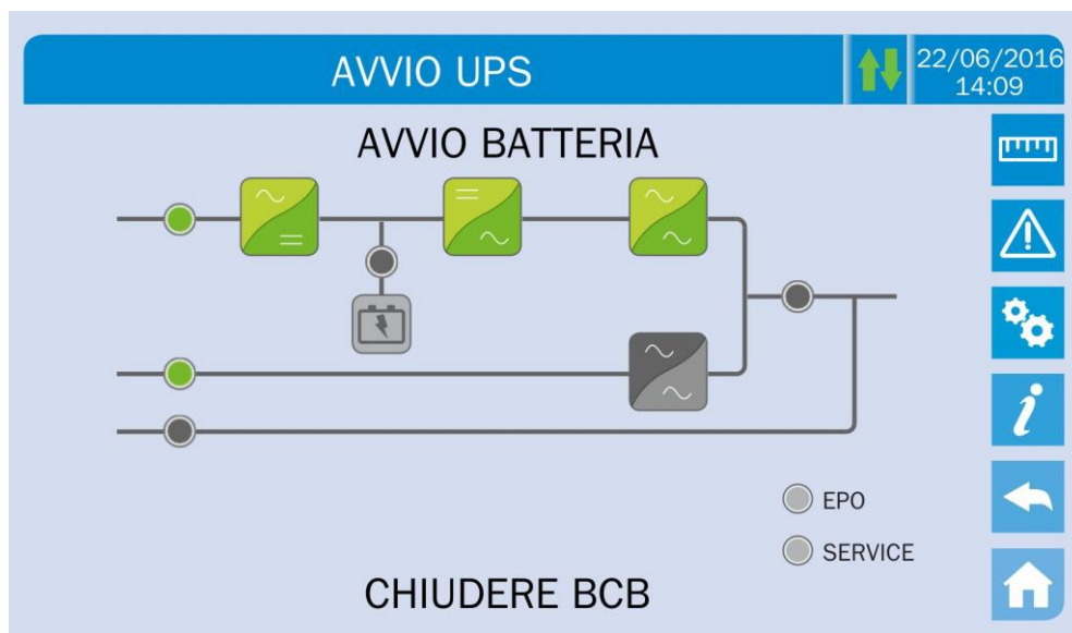
Figura 14 – Avvio batteria
