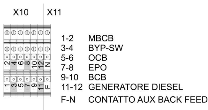
Figura 7 – Morsetti ausiliari KEOR HPE 200-250-300 kVA
