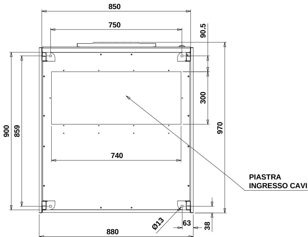
Figura 3 – Pianta di base
