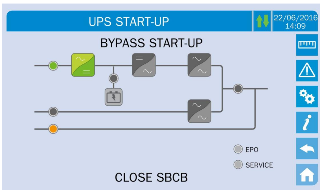
Illustration 18 – Départ différé
