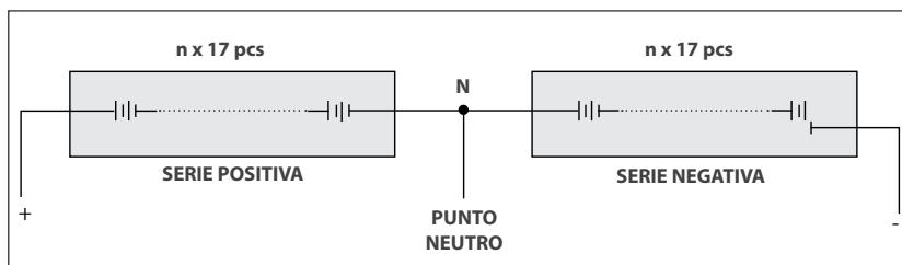
Dos grupos en serie con punto central – Potencial neutro –
