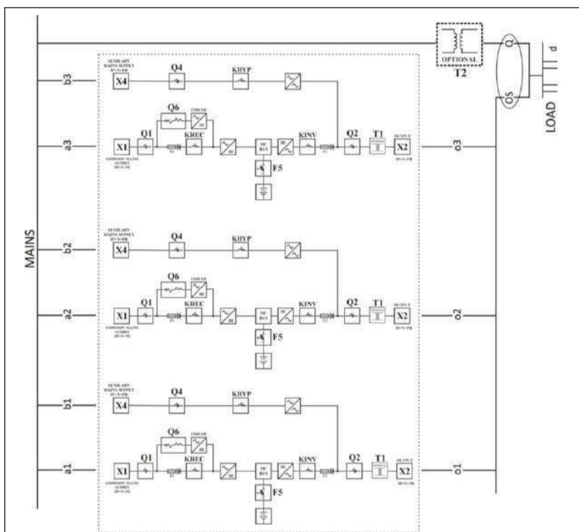
TRES UNIDADES EN PARALELO Configuración redundante N+1 con entrada de distribución doble
