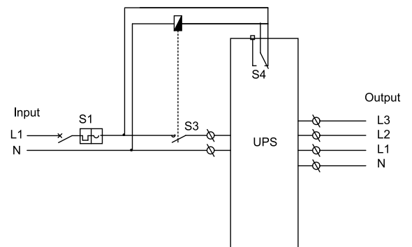
Configuração Mono-fásica/Tri-fásica
