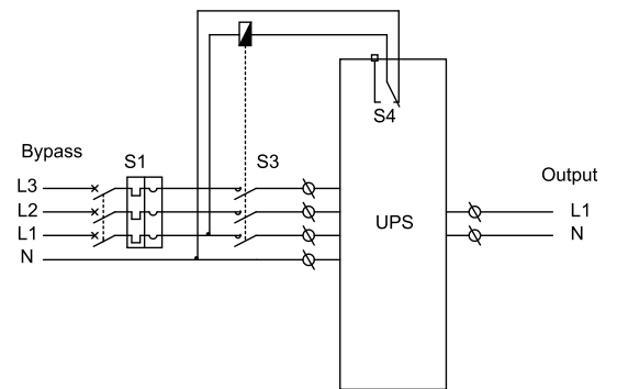
Configuração Tri-fásica/Mono-fásica
