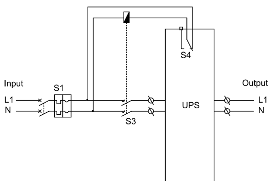
Configuração Mono-fásica/Mono-fásica
