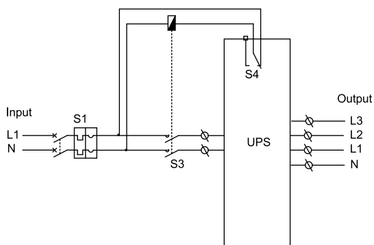
Configuração Mono-fásica/Tri-fásica
