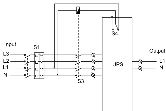
Configuração Tri-fásica/Mono-fásica
