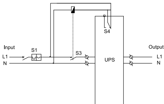
Configuração Mono-fásica/Mono-fásica
