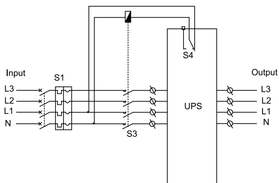
Configuração Tri-fásica/Tri-fásica
