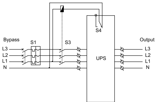
Configuração Tri-fásica/Tri-fásica
